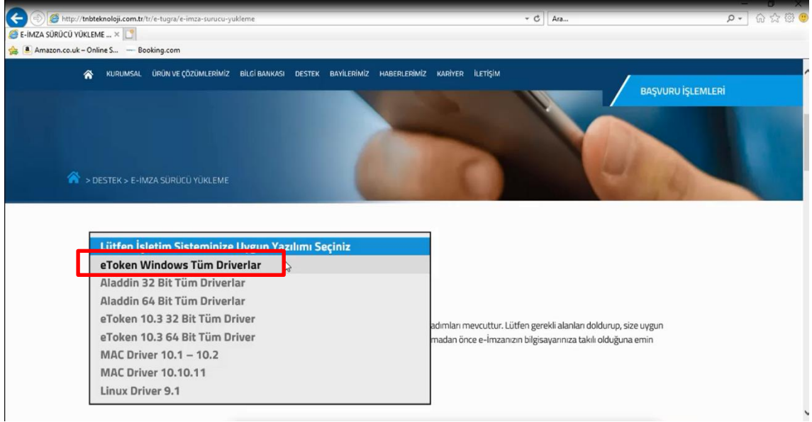
Şekil 3: Driver seçimi
