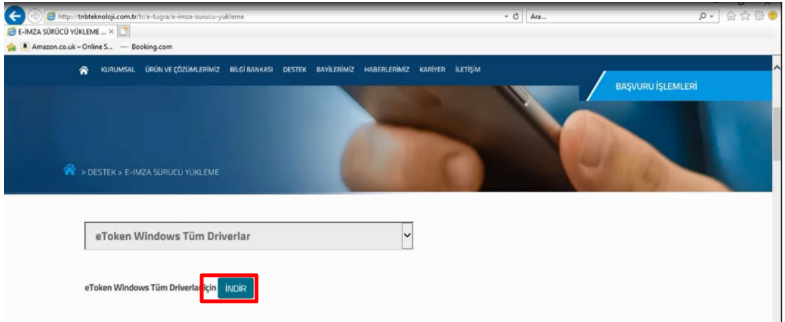
Şekil 4: İndirme düğmesi
